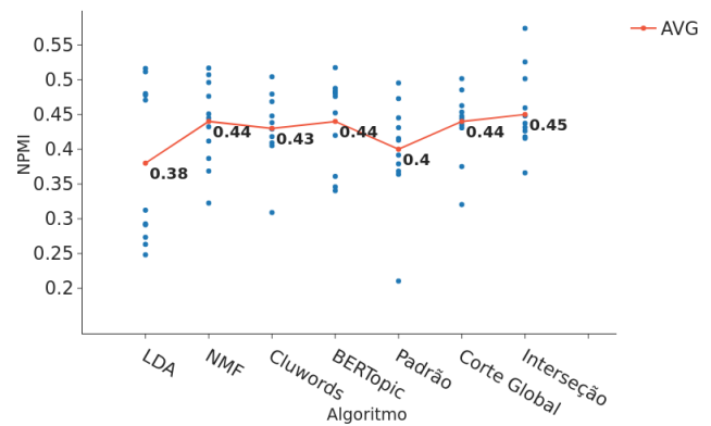
Figura 3. Valores de NPMI para diferentes algoritmos na base ACM.
