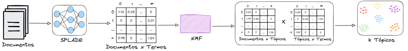
Figura 1. Pipeline de modelagem de tópicos.
