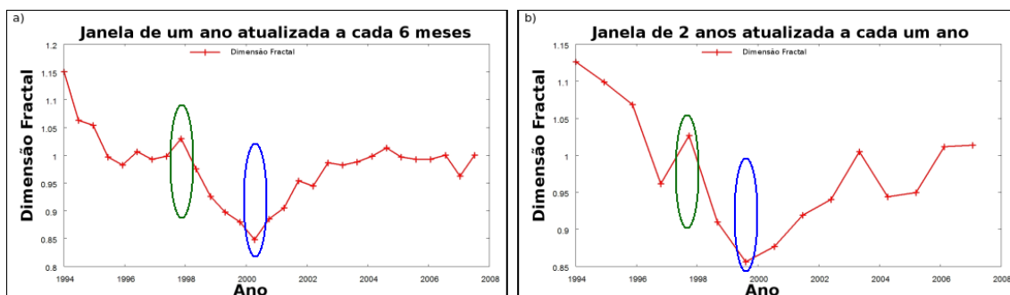
Figura 5. Variação de D_2 para a região Sul: (a) janela de um ano com deslocamento de 6 meses; (b) janela de 2 anos com deslocamento de um ano.
