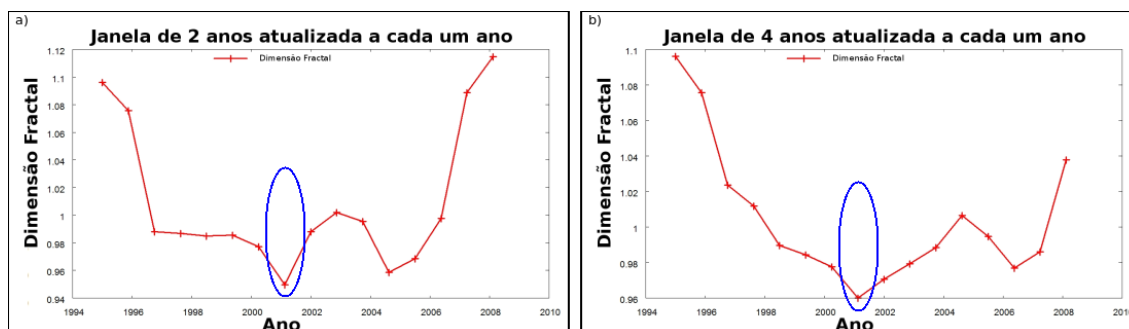
Figura 6. Variação de D_2 para o estado de São Paulo: (a) janela de 2 anos com deslocamento de um ano; (b) janela de 4 anos com deslocamento de um ano.
