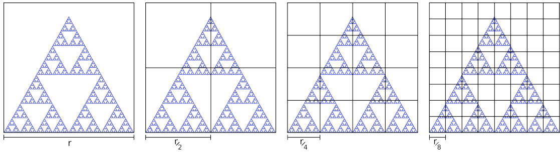
Figura 1. Variação de r das células que compõem um hiper-reticulado de duas dimensões que dividem um triângulo de Sierpinski.
