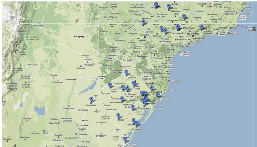
Figura 4. Localização das estações meteorológicas - SP e região Sul.
