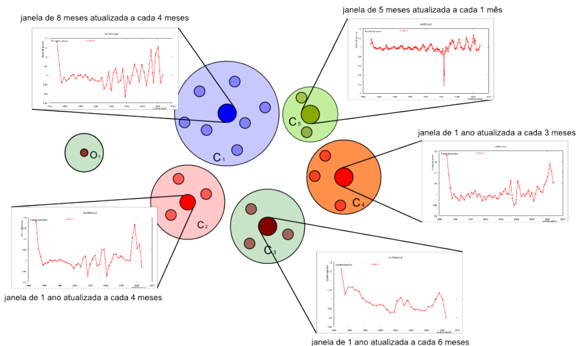
Figura 7. Grupos de gráficos D_2 para São Paulo (C - grupos e O - extremos).
