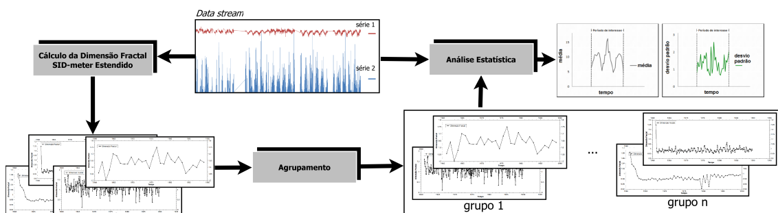
Figura 3. Processo de análise de múltiplas séries temporais.
