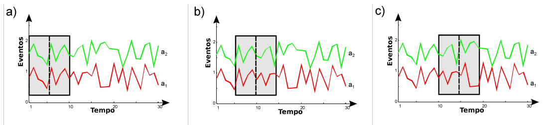
Figura 2. Janela deslizante sobre uma data stream bi-dimensional.
